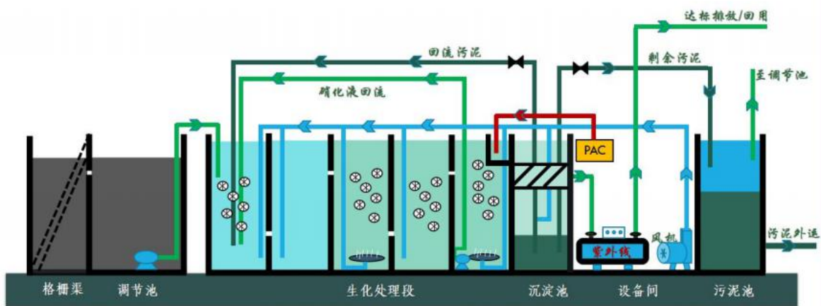
图 4 MSC-MBBR 工艺原理图
