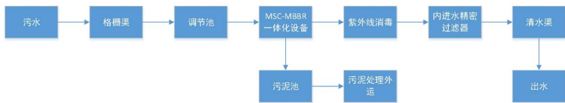
图 3 本工程工艺流程图
